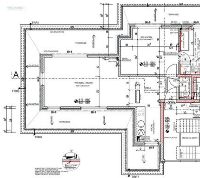
Grundriss
